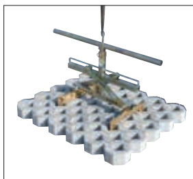
Chwytek TSV z adapterem do układania płyt ażurowych
