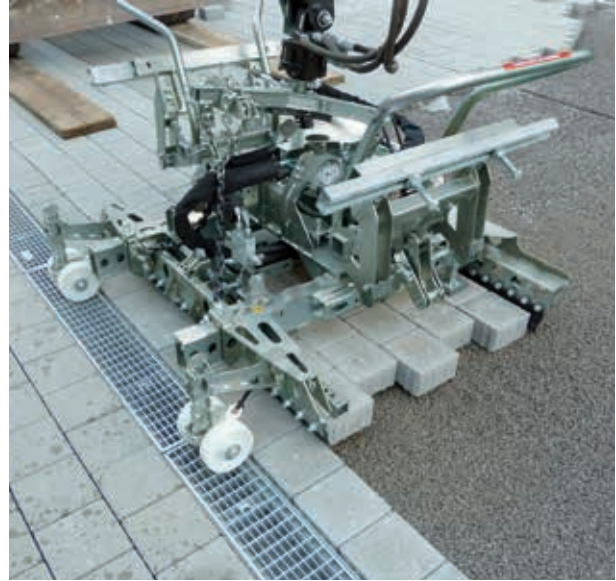
HVZ-ECO Chwytnak hydrauliczny do układania kostki
